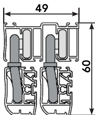
Coupe verticale
