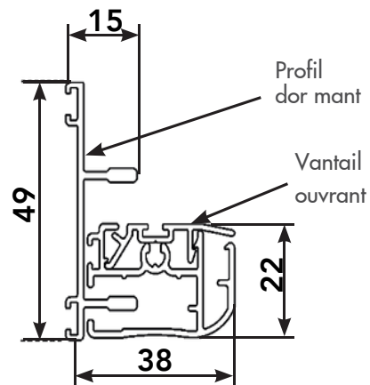
Coupe horizontale
