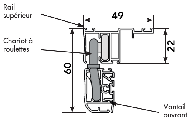
Coupe verticale
