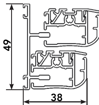
Coupe horizontale
