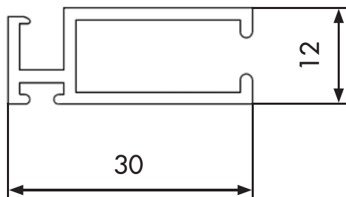
Profil aluminium
