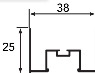
Coupe du profil (pose ou réception)
