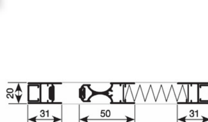
Coupe horizontale
