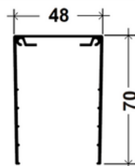
Profil supérieur
