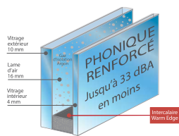
28 mm - 10/14/4 Faiblement émissif avec gaz argon Coefficient d'affaiblissement acoustique jusqu'à 33dBA Coefficient thermique Ug : 1.1 W/ m 2 K
