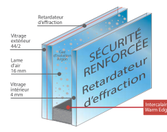
28 mm - 44.2/14/4 Faiblement émissif avec gaz argon Retardateur d'effraction Coefficient thermique Ug : 1.1 W/ m 2 K
