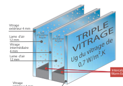
36 mm - 4/12/4/12/4 Faiblement émissif avec gaz argon Deux couches de gaz argon entre chaque lame de verre. Isolation optimale (option indisponible pour les fenêtres à ouvrant caché) Coefficient thermique Ug : 0.7 W/ m 2 K
